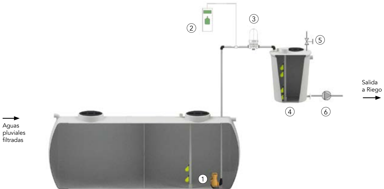
DEPÓSITO DE ALMACENAMIENTO DE AGUAS PLUVIALES
