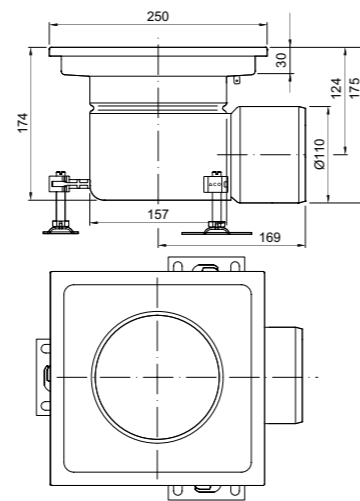
EG Fijo 250x250mm DN110 Salida Horizontal Saída Horizontal
