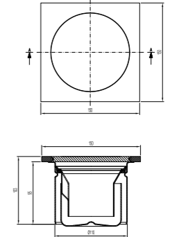
Sumidero EG150 Estanco Sumidouro EG150 Estanque
