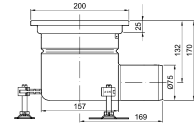
EG Fijo 200x200mm DN75 Salida Horizontal Saída Horizontal
