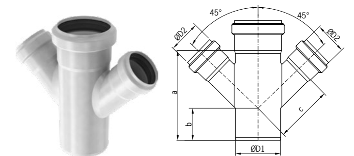
Derivación doble con reducción 45° Derivação suplo 45° com redução
