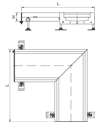
Canal de esquina Canal de canto
