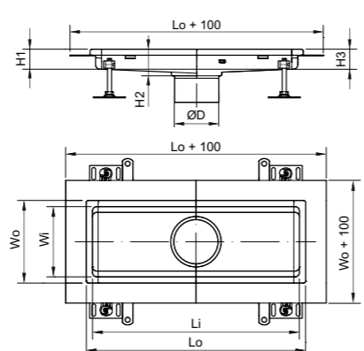
Canal ACO Box Semi-Estándar · Perfil extendido Canal ACO Box Semi-Standard · Perfil estendido
