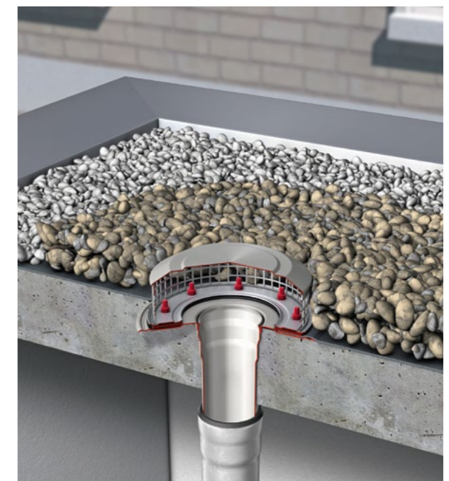
Sumidero de cubierta de acero inoxidable con brida para clipaje por compresión Sumidouro de cobertura de aço inoxidável com flange para clipagem por compressão
