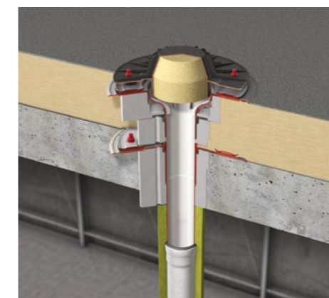
Sumidero de acero inoxidable con dos bridas de clipaje por compresión Sumidouro de aço inoxidável com duas flanges de clipagem por compressão
