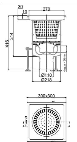
EG con Cestillo Extendido Fijo com Cesto Estendido Fixo 300x300mm DN110 Salida Vertical Saída Vertical
