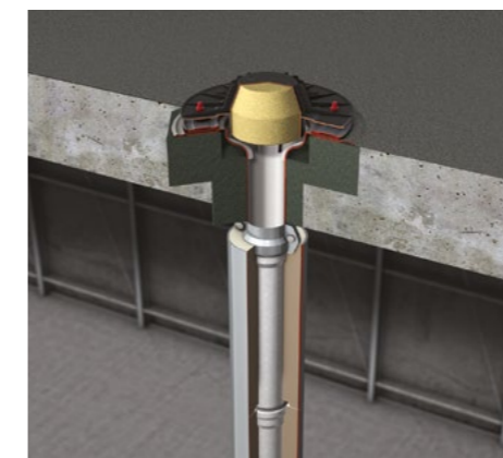
Sumidero de cubierta Jet de acero inoxidable con brida de clipaje por compresión Sumidouro de cobertura Jet de aço inoxidável com flange de clipagem por compressão
