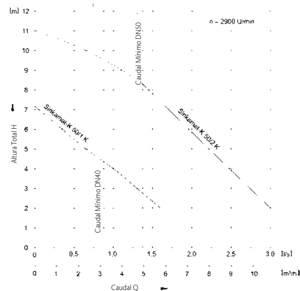
Caudal Flujo Q - Altura manométrica H
