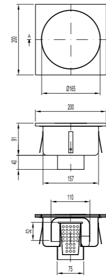
Sumidero Sifónico Select 200x200 Estanco Sumidouro Sifónico Select 200x200 Estanque
