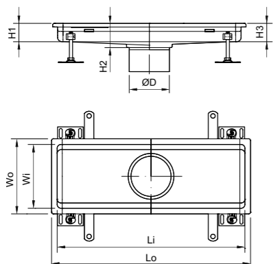
Canal ACO Box Semi-Estándar · Perfil Estándar Canal ACO Box Semi-Standard · Perfil Standard
