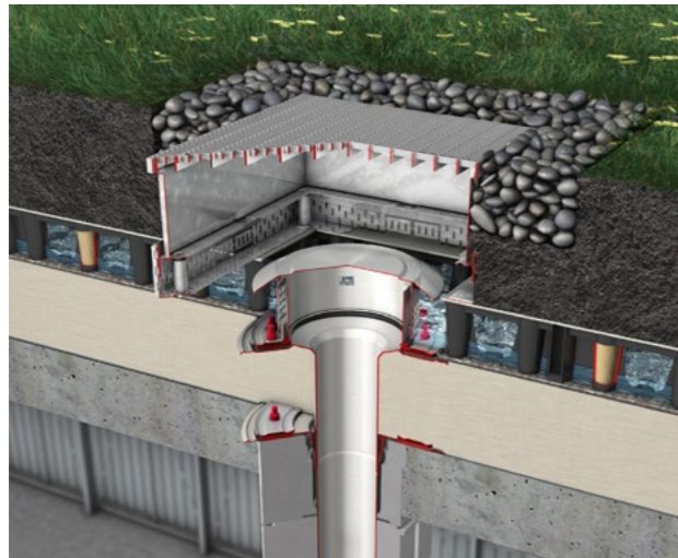
Cubierta verde con drenaje y accesorio de retención. Cobertura verde com drenagem e acessório de retenção.
