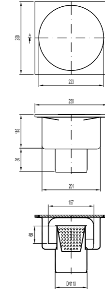
Sumidero Sifónico Select 250x250 Estanco Sumidouro Sifónico Select 250x250 Estanque
