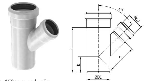
Derivación simple con reducción 45° Derivação simple 45° com redução
