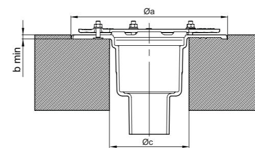
Representación con accesorios contra incendios.
