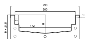
Canal Modular CM200 Canal Modular CM200
