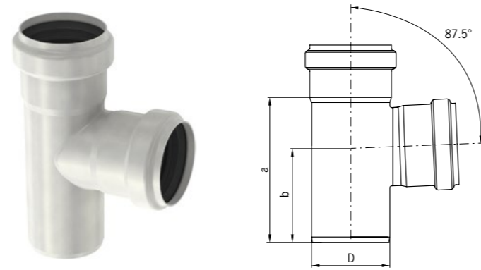
Derivación simple 87,5° Derivação simple 87,5°
