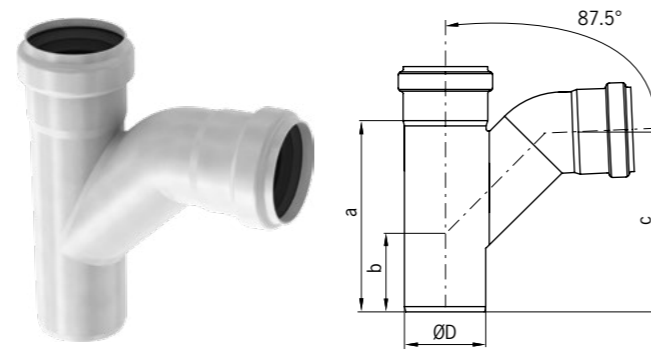
Derivación simple con codo 45° Derivação simple com curva 45°
