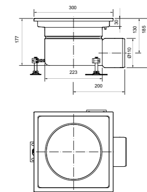
Sumidero EG250 Estanco S/H Sumidouro EG250 Estanque S/H
