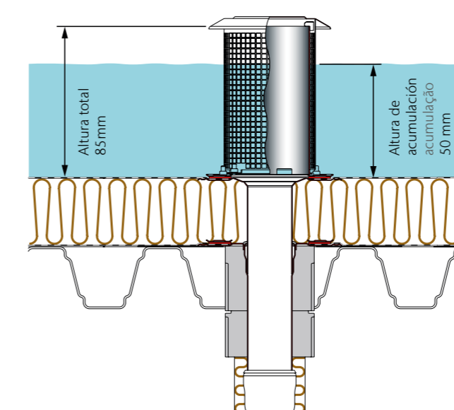
Evacuación de agua con elemento de retención Evacuação da água com elemento de retenção
