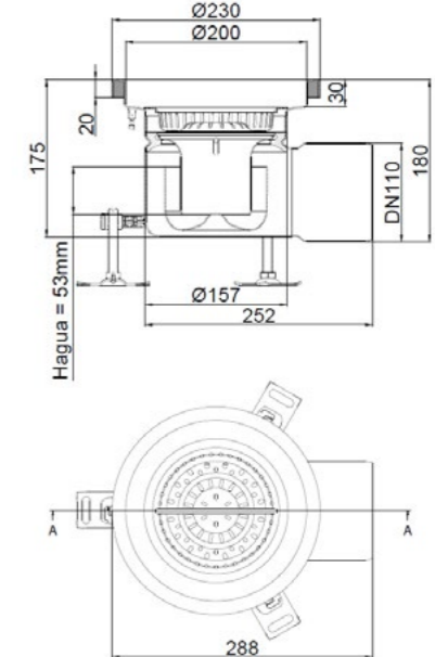
EG Fijo Fixo ø230mm DN110 Salida Horizontal Saída Horizontal
