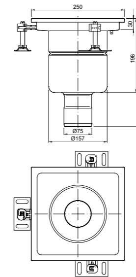
EG Fijo 200x200mm DN75 Salida Vertical Saída Vertical
