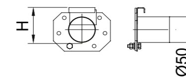
Tapa Final con Salida DN50 Tampa de final com Saída DN50
