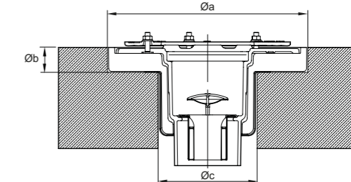
Representação com acessórios contra fogo.
