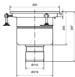
Sumidero EG300 Estanco S/V Sumidouro EG300 Estanque S/V
