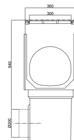
Plano sumidero Elementos técnicos do sumidouro
