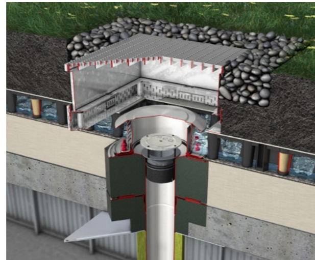
Cubierta verde con drenaje, accesorio de retención e inserto antiincendios. Cobertura verde com drenagem, acessórios de retenção e inserto anti-incêndio
