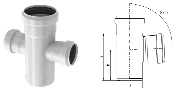
Derivación doble con reducción 87,5° Derivação duplo 87,5° com redução
