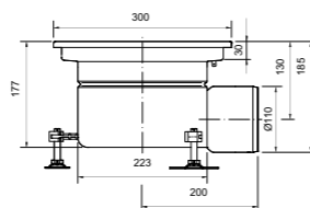
Sumidero EG300 Estanco S/H Sumidouro EG300 Estanque S/H
