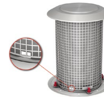
Elemento de retención para cubierta DN 70/DN 100 Elemento de retenção para cobertura DN 70/DN 100
