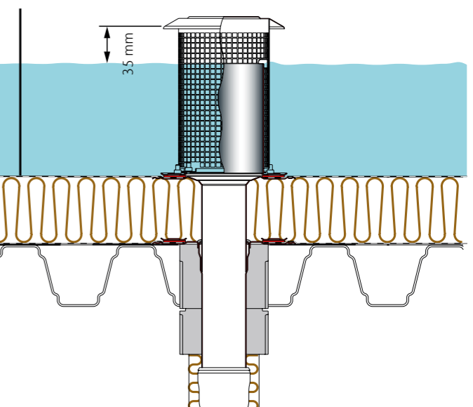
Elemento de retenção para la evacuación de agua de emergencia Elemento de retenção para a evacuação de água de emergência
