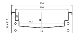
Canal SIN pendiente Canal SEM pendiente
