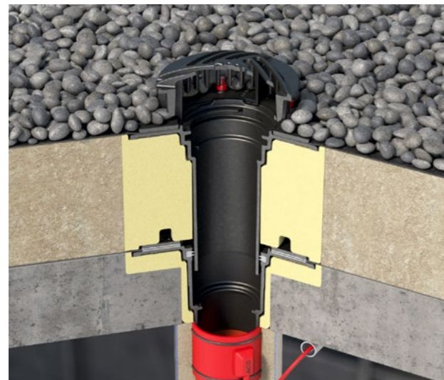
Sumidero de cubierta ACO de hierro fundido con doble clipaje mecánico Sumidouro de cobertura ACO de fundição com clipagem mecânica dupla.
