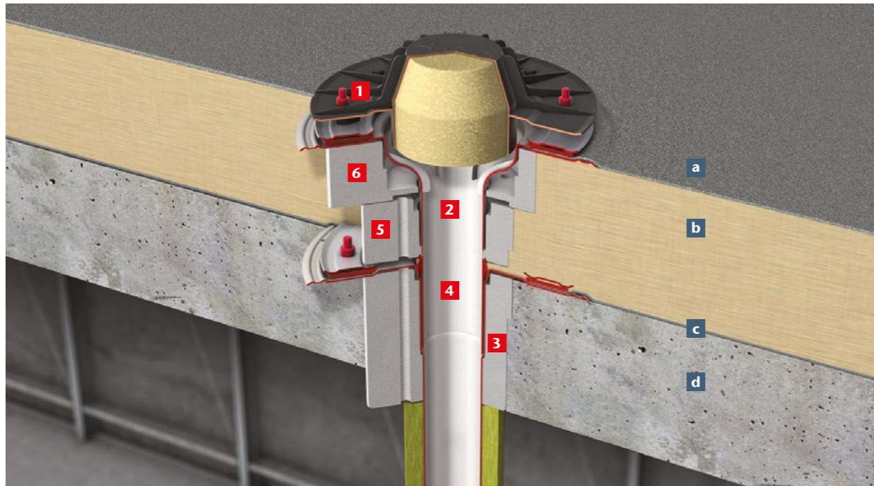
Sumidero completo, Código. 12792500, compuesto de: Sumidouro completo, Código 12792500, composto de:
