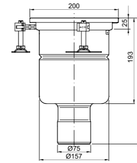
EG Fijo 200x200mm DN75 Salida Vertical Saída Vertical
