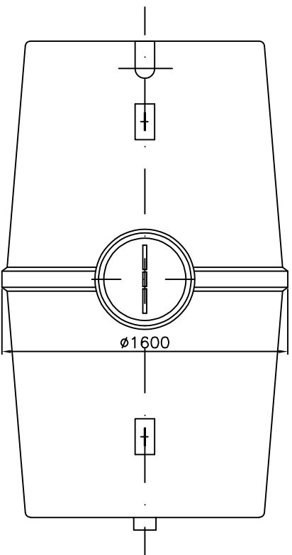
DETALLE OREJA DE ELEVACION TIPO DE OREJAS: MONTAJE 2
