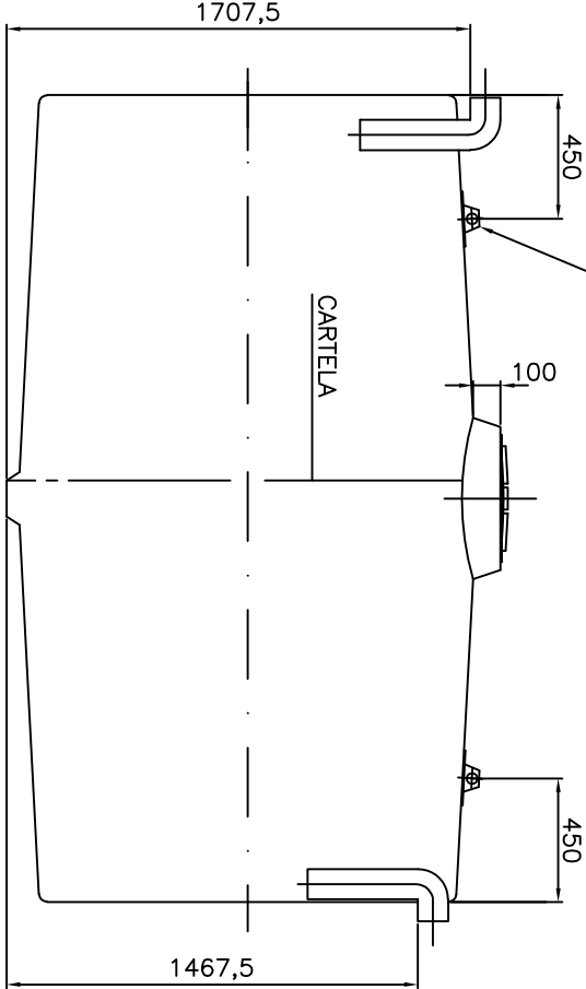
OREJAS TIPO MONTAJE 2
