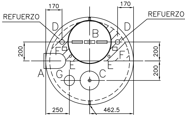
DETALLE OREJA DE ELEVACIÓN TIPO DE OREJAS: OMEGA
