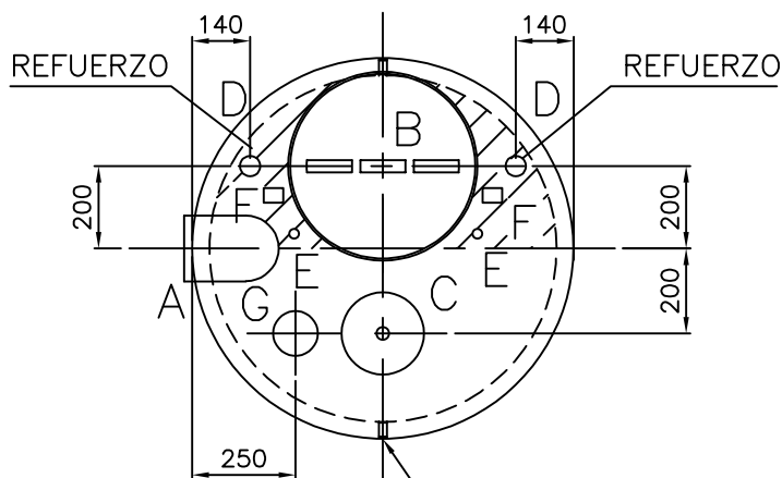
DETALLE OREJA DE ELEVACIÓN TIPO DE OREJAS: OMEGA
